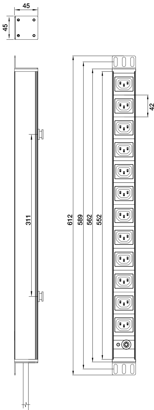
15A Standard Mains
